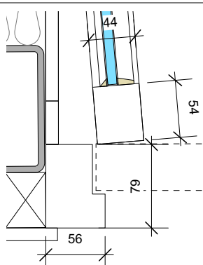
Door ID07 1:5 Plan detail Jamb
