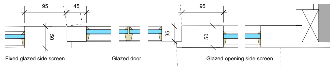
Door ID10 1:5 Plan details
