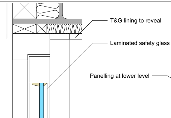
Door ID07 1:5 Section detail Head
