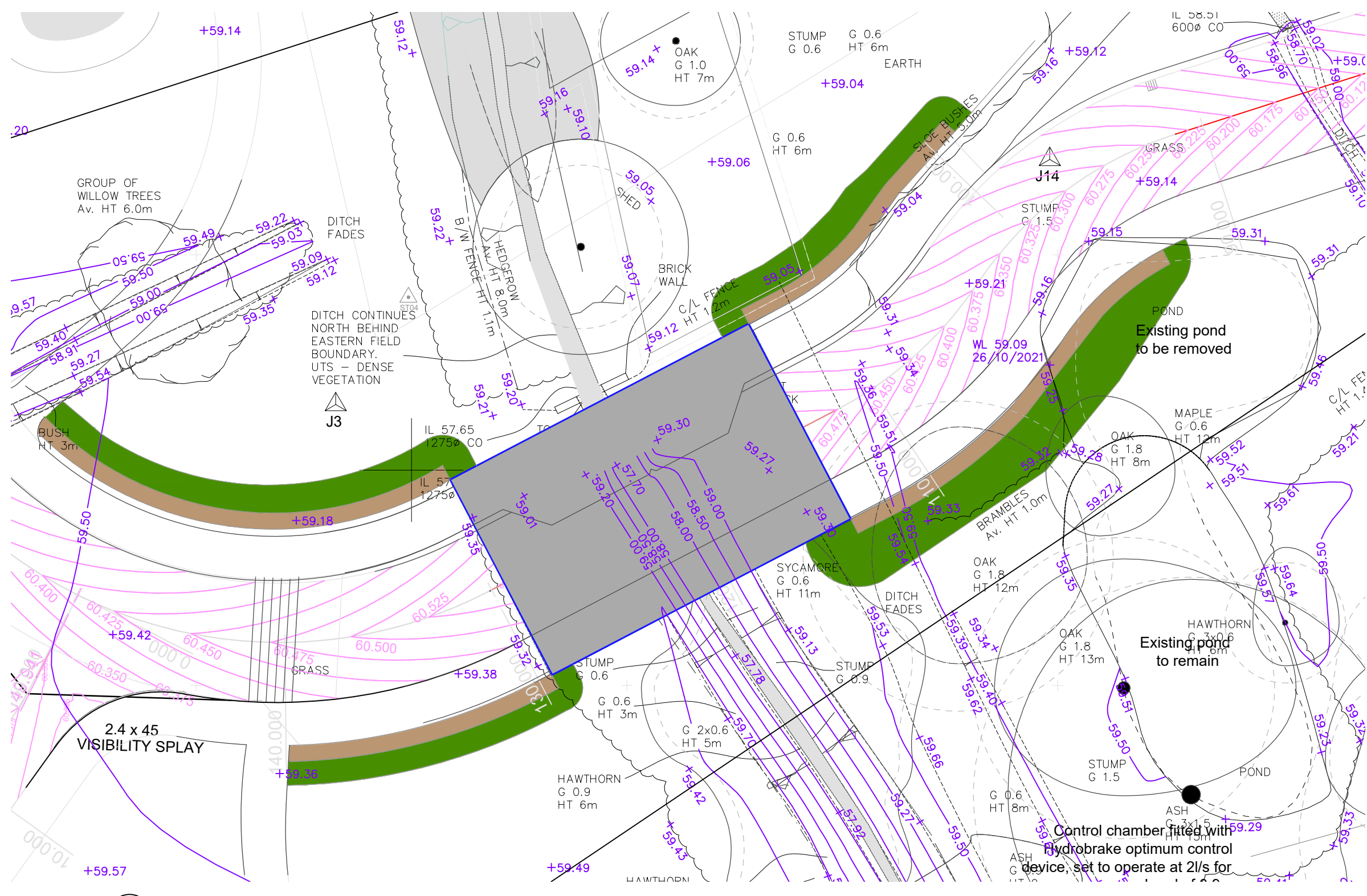
SITE PLAN 1:200
