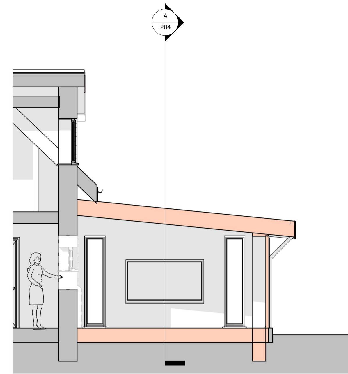
Section B 1 : 50
