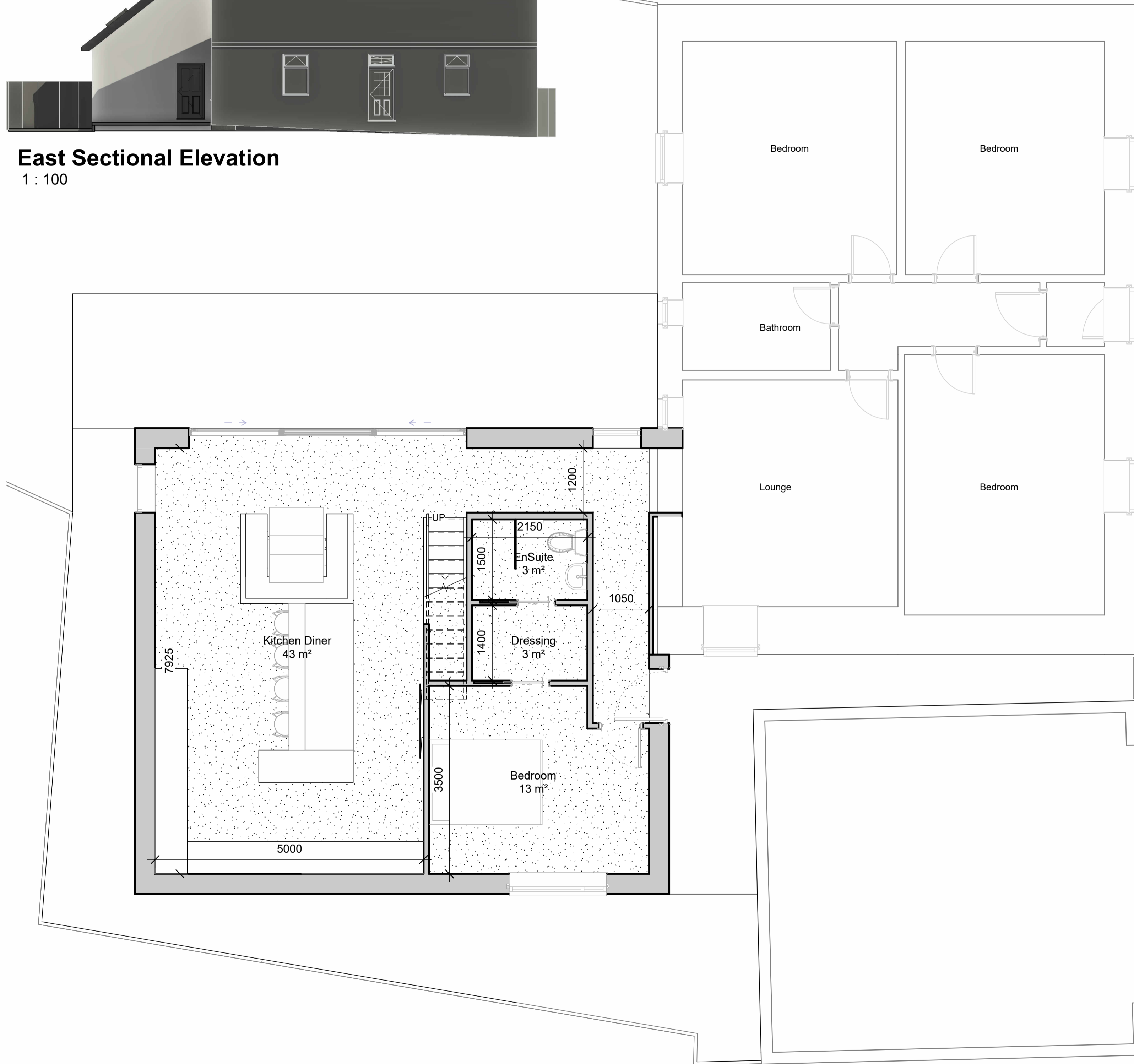
GF Ext 1 : 50
