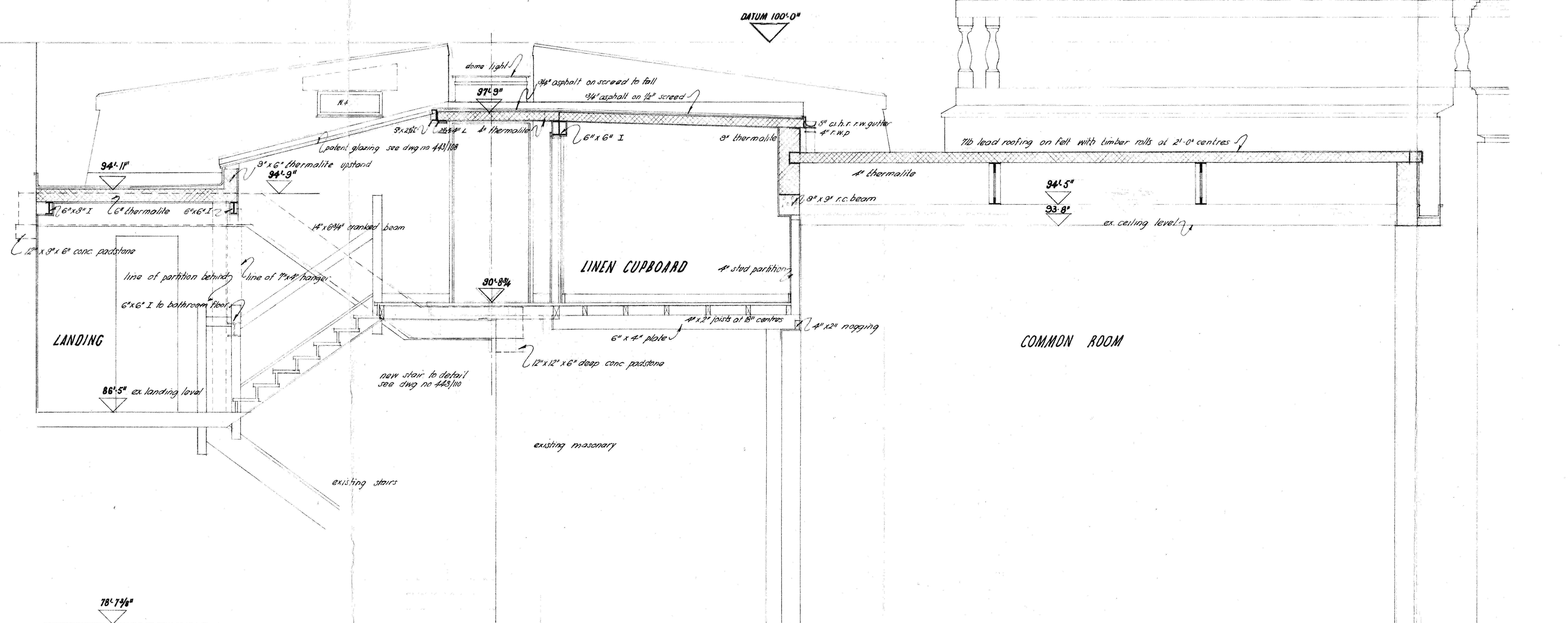
SECTION A-A
