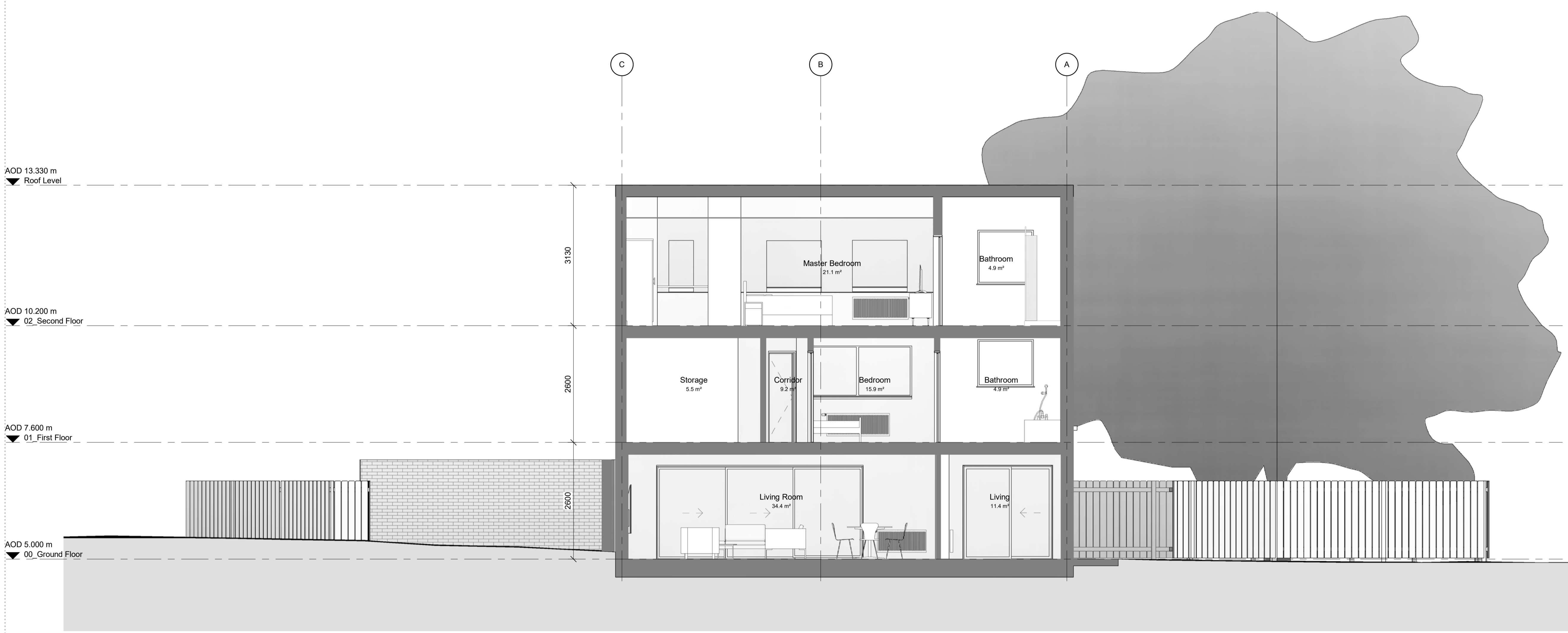
1 Existing Section B-B 20301 1 : 50
