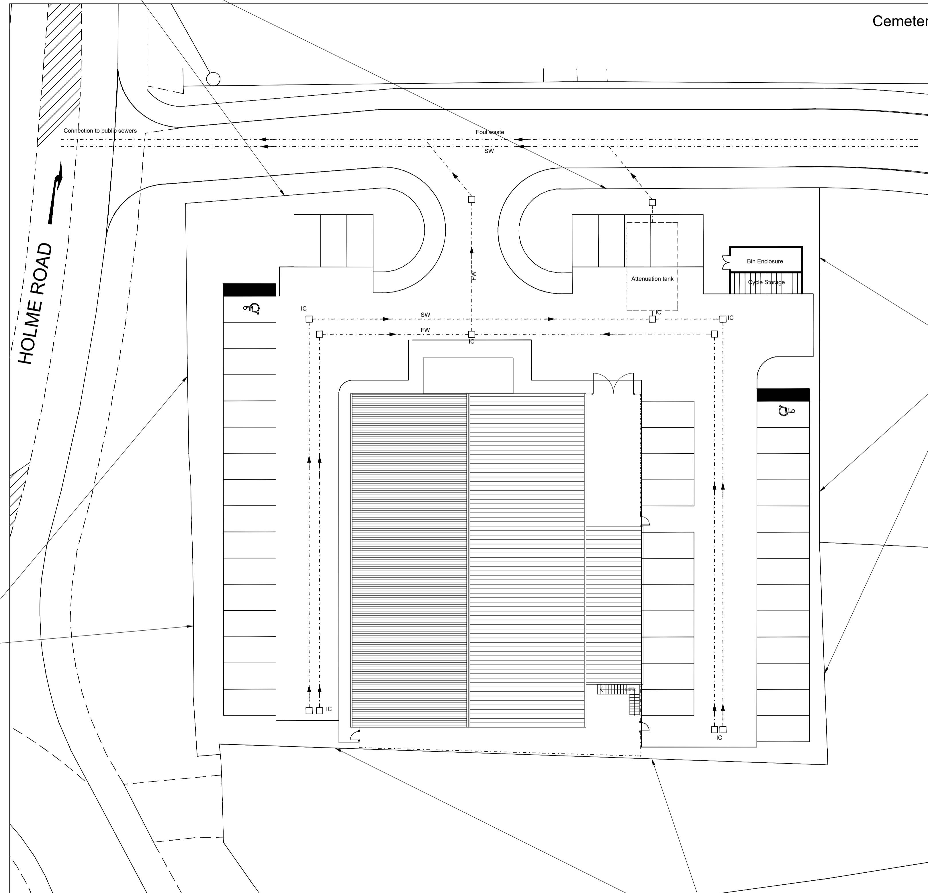
02 EXISTING SITE PLAN 1:200
