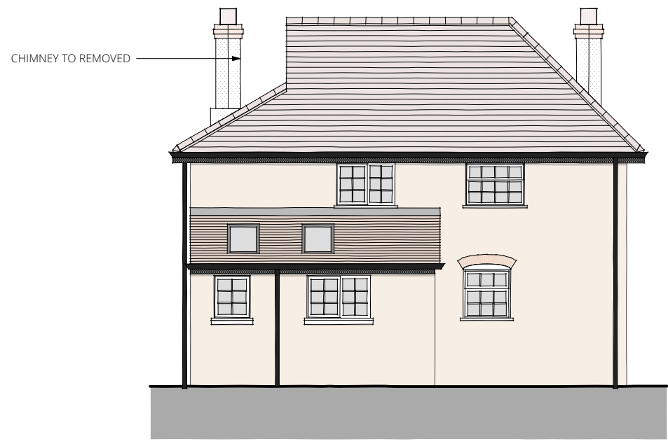
ELEVATION 02
