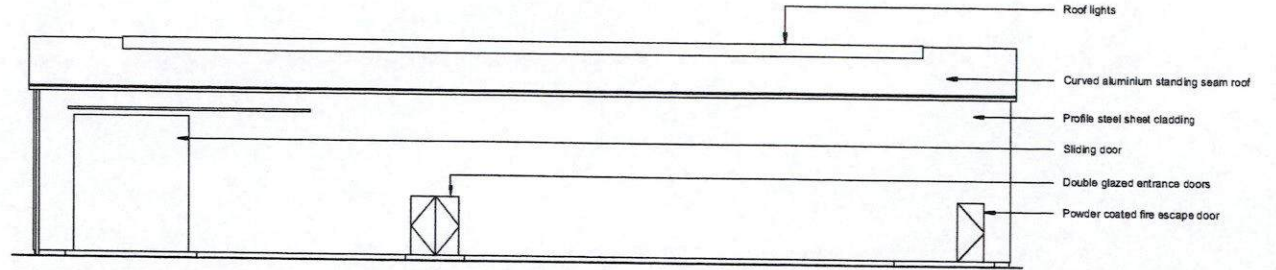
Elevation A
