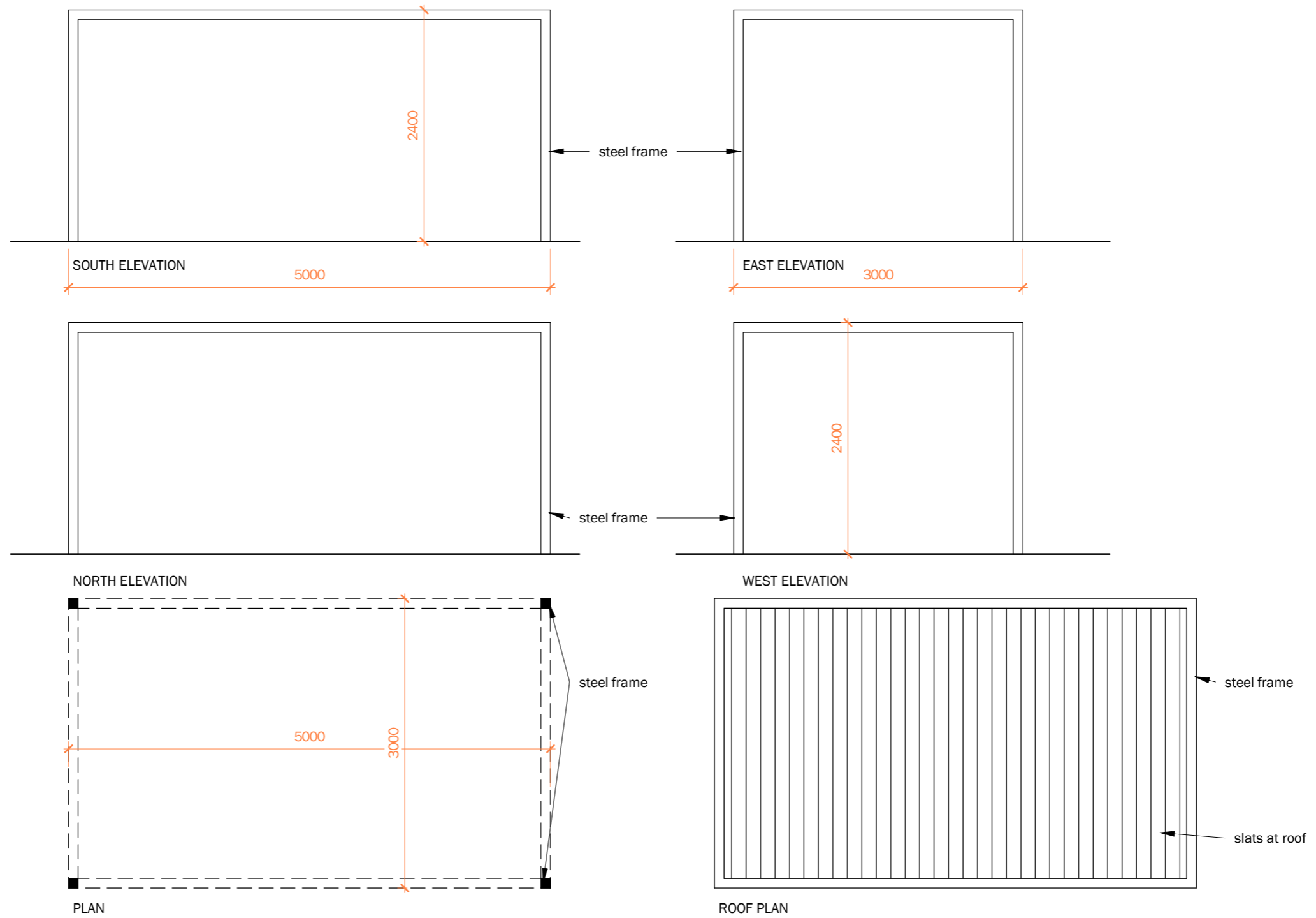
Pergola 1 1 : 50
