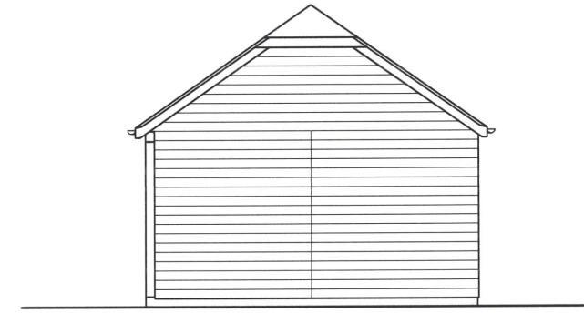
Right Elevation
