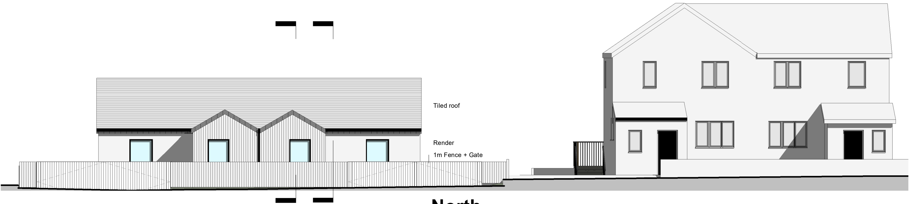
North 1 : 100
