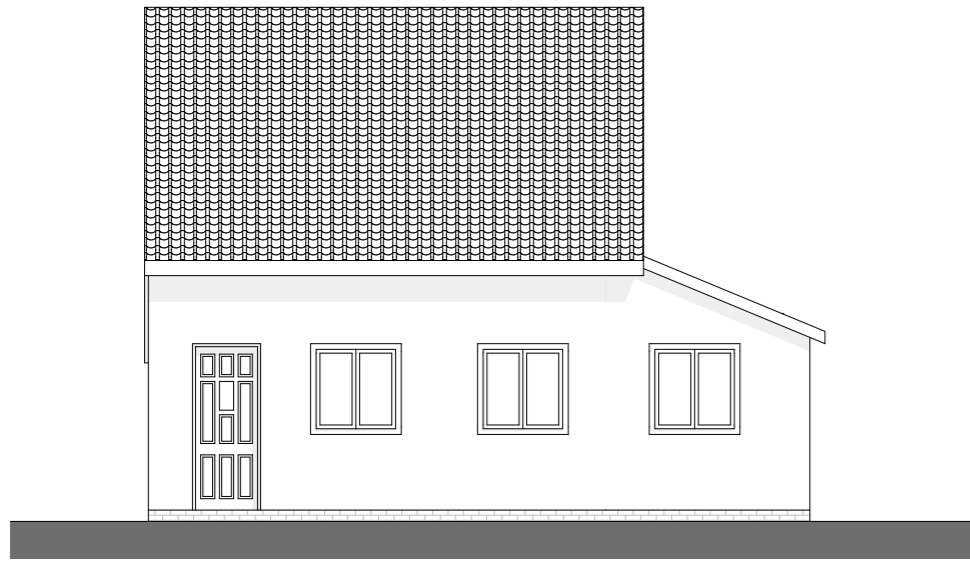
1:100 E1 Front Elevation
