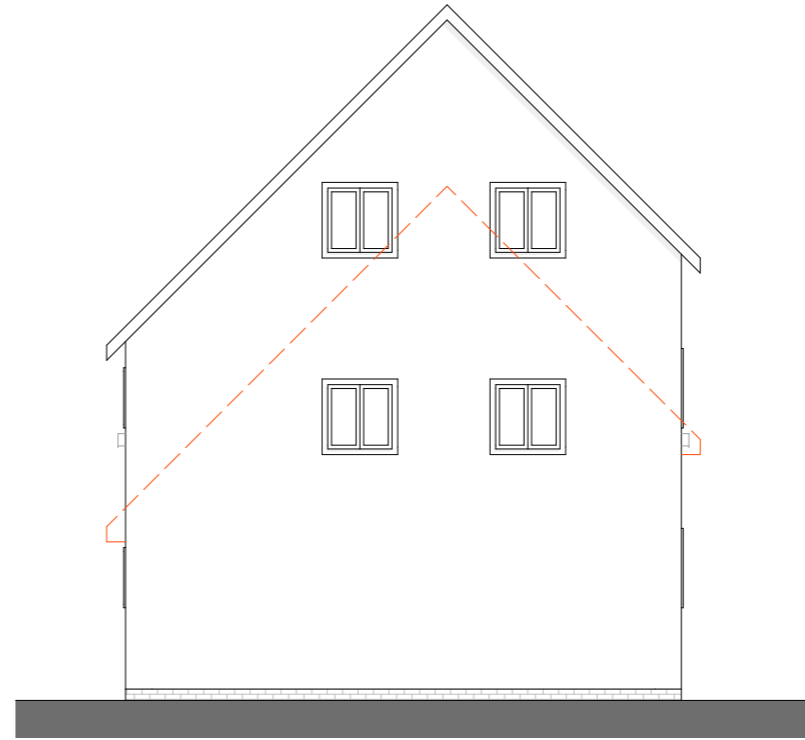
1:100 E10 Side Elevation
