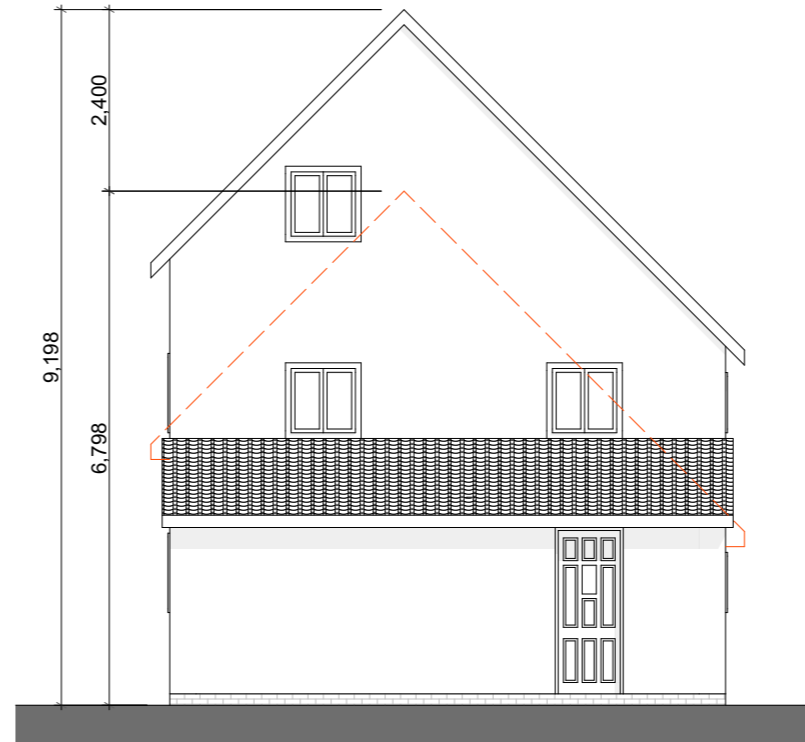
1:100 E12 Side Elevation
