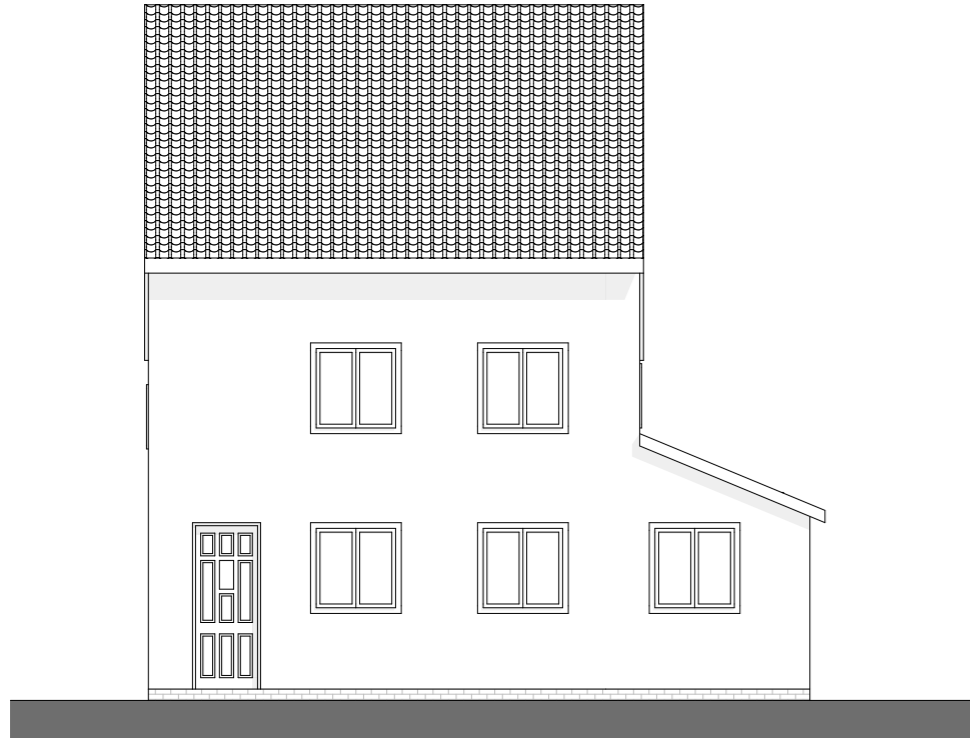
1:100 E9 Front Elevation
