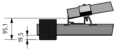
A ( 1 : 10 )
