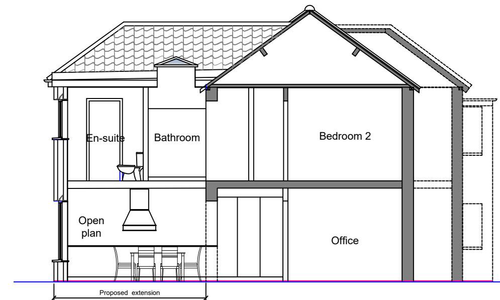
Section A-A 1:100
