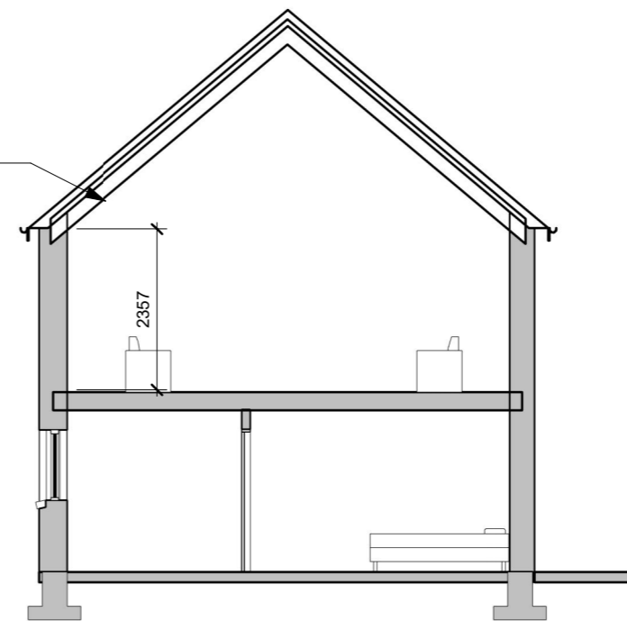
Section thru lounge 1 : 100
