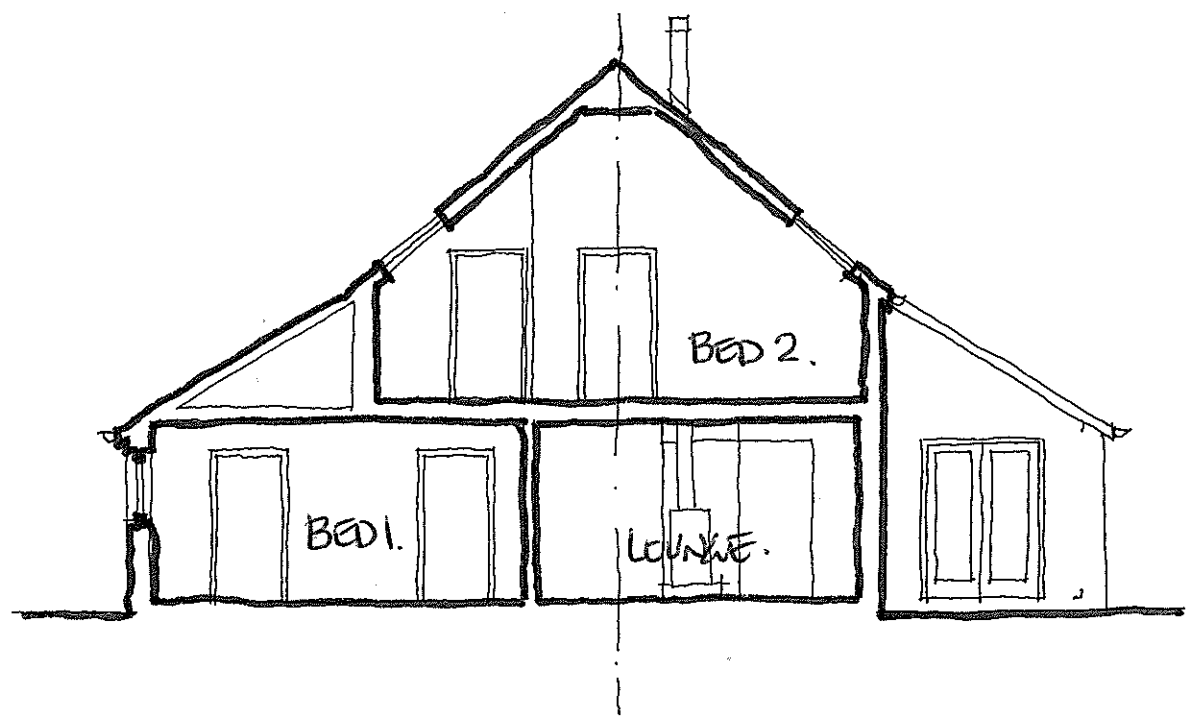
SECTION A-A 1:100 @ A3
