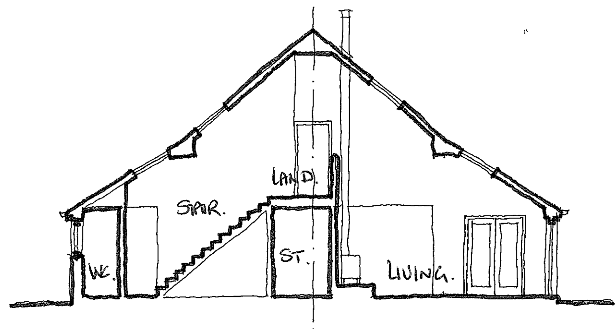
SECTION B-B 1:100 @ A3
