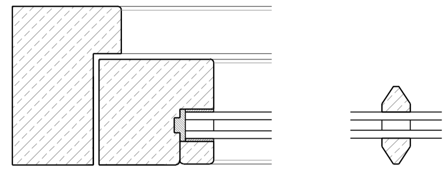
Horizontal Window Section - Scale: 1:2
