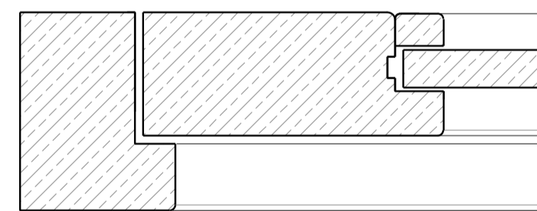
Lower Horizontal Door Section - Scale: 1:2
