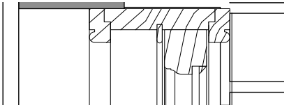
SECTION DETAIL DOOR 1:5
