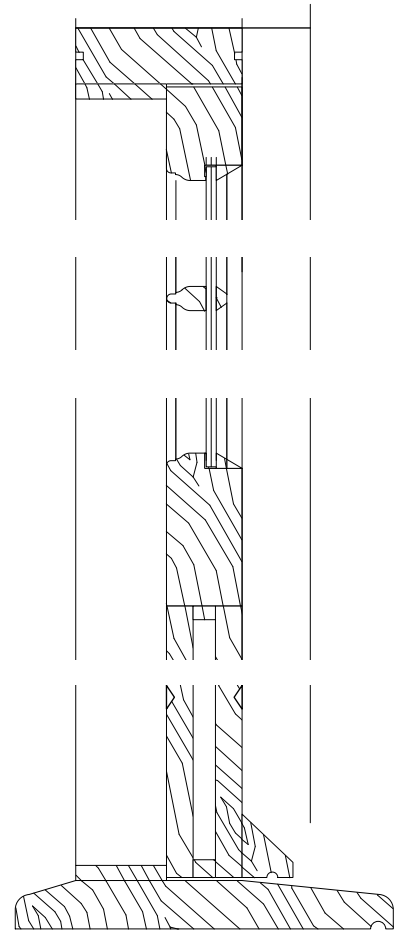
SECTION DETAIL DOOR 1:5
