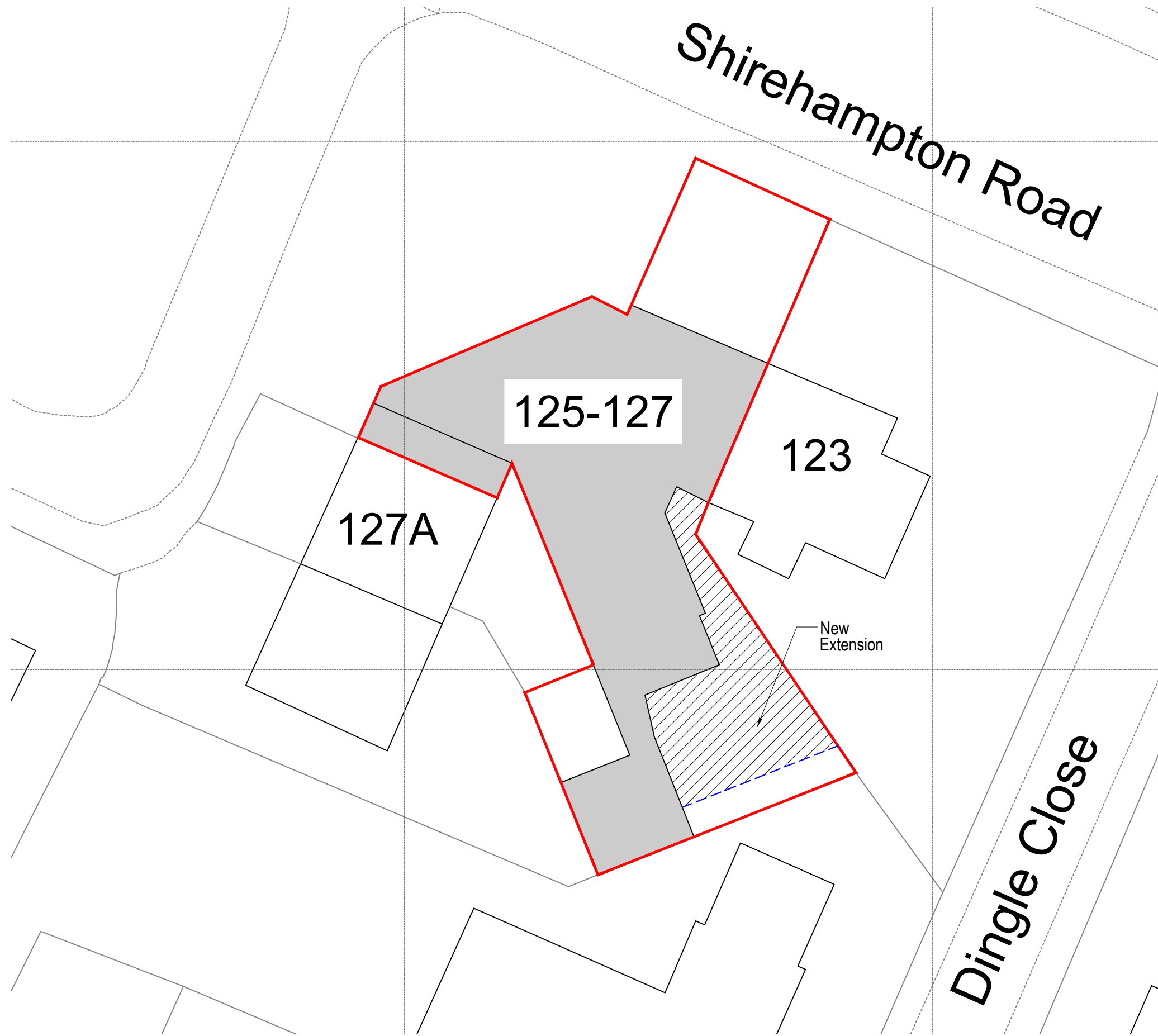
Site plan (1:200)
