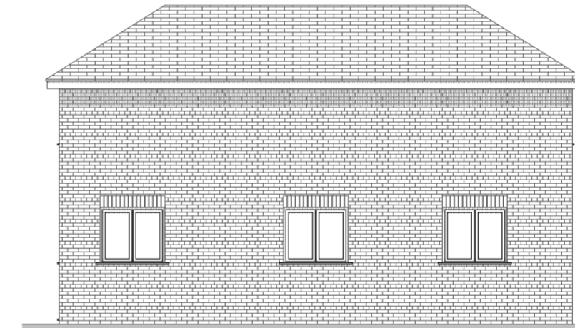
E-06 E 1:100
