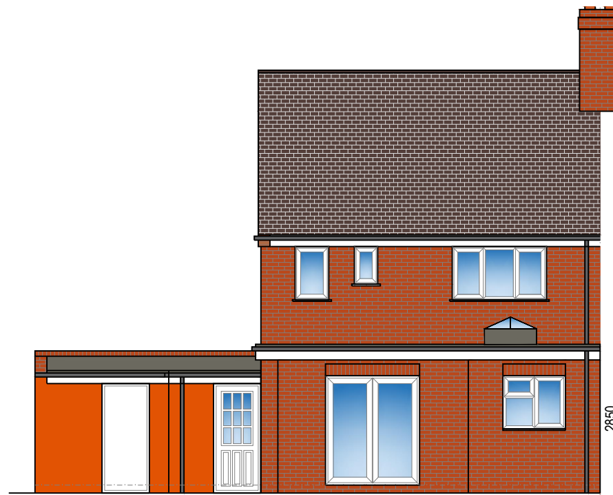
R E A R E L E V A T I O N
