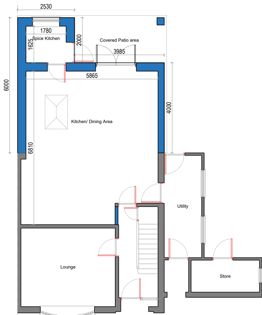
G R O U N D F L O O R P L A N
