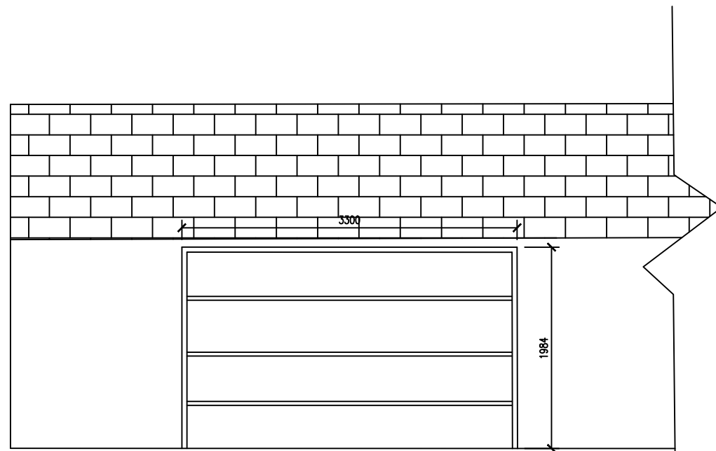
Existing Door 1:50
