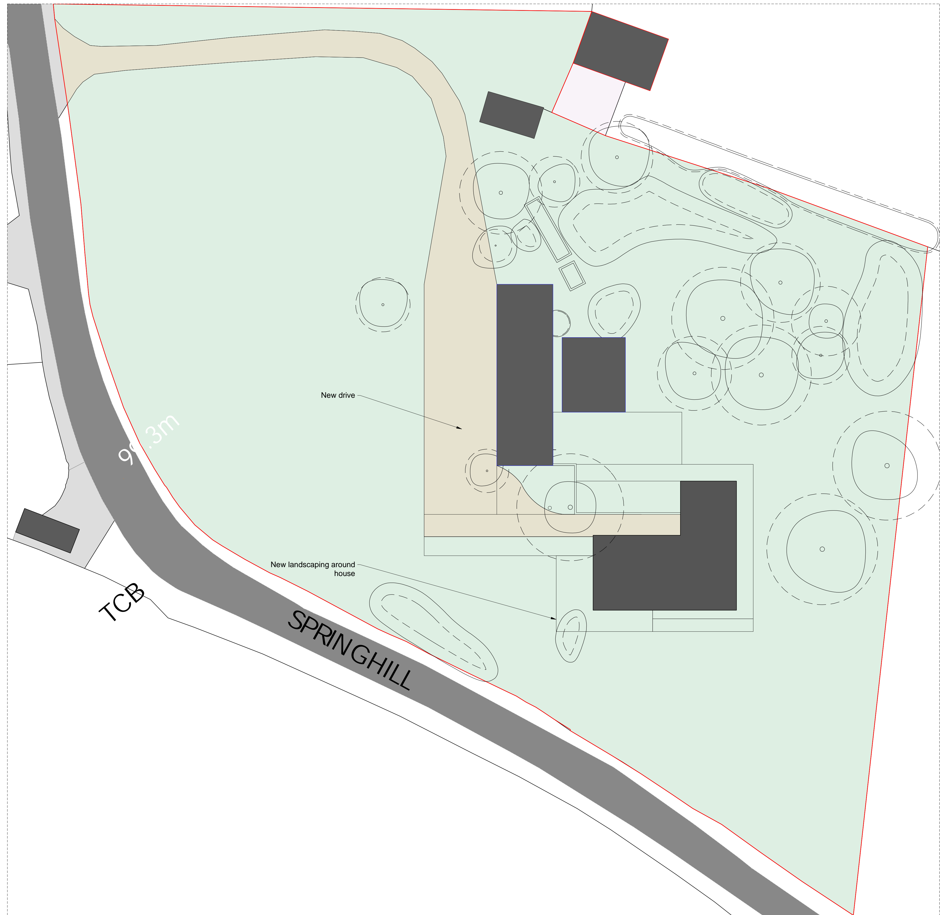
1 EXISTING LANDSCAPE Scale: 1:200
