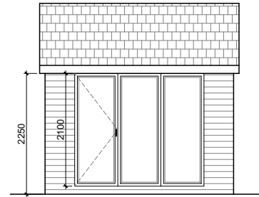
LEFT ELEVATION SCALE 1:100 @A4
