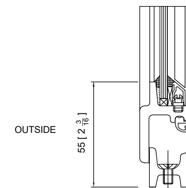
JAMB DETAIL
