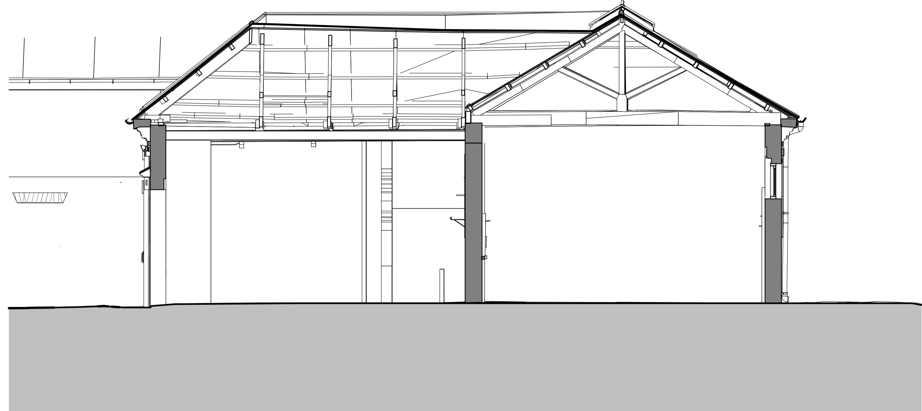
Section 10 - Existing 1 : 50
