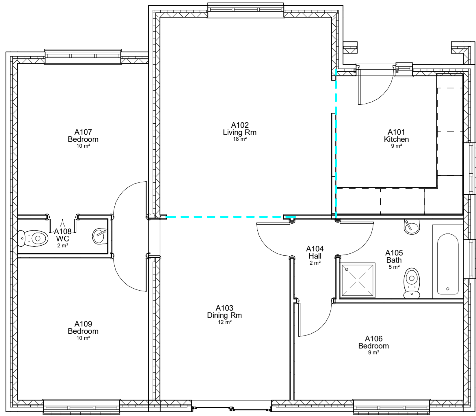
1 Existing FFL 1 : 50
