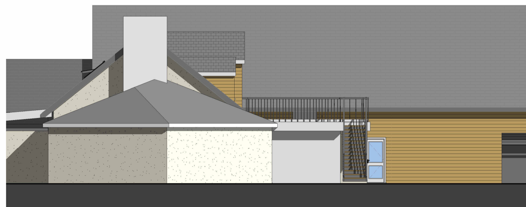
1 East 1 : 100
