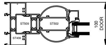
08 DOOR JAMB DETAIL
