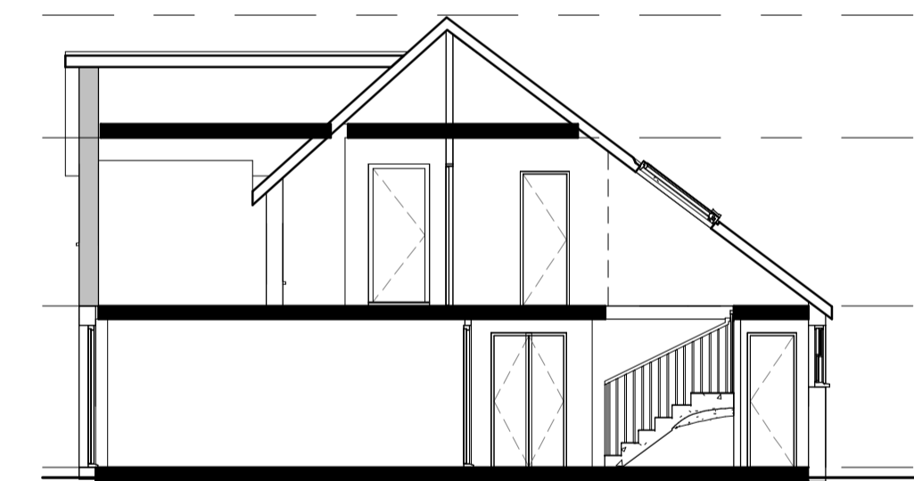
15 Section xy 1 : 100
