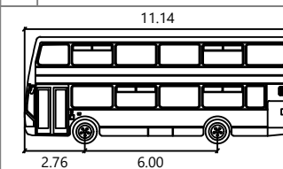
2018 Optare Metrodecker MD11140
