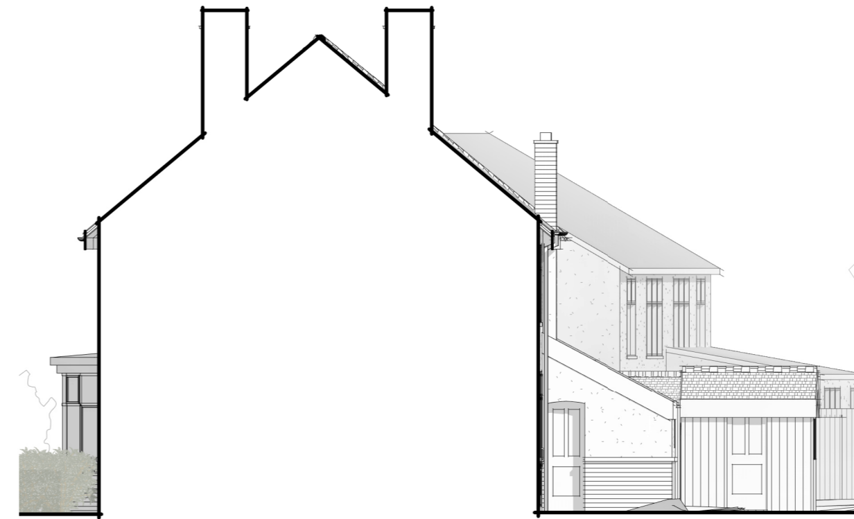
6 | Side Elevation 2 1 : 100 | A-101
