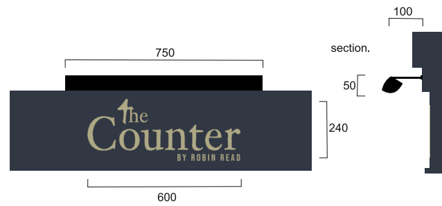
1:20 @ A3
