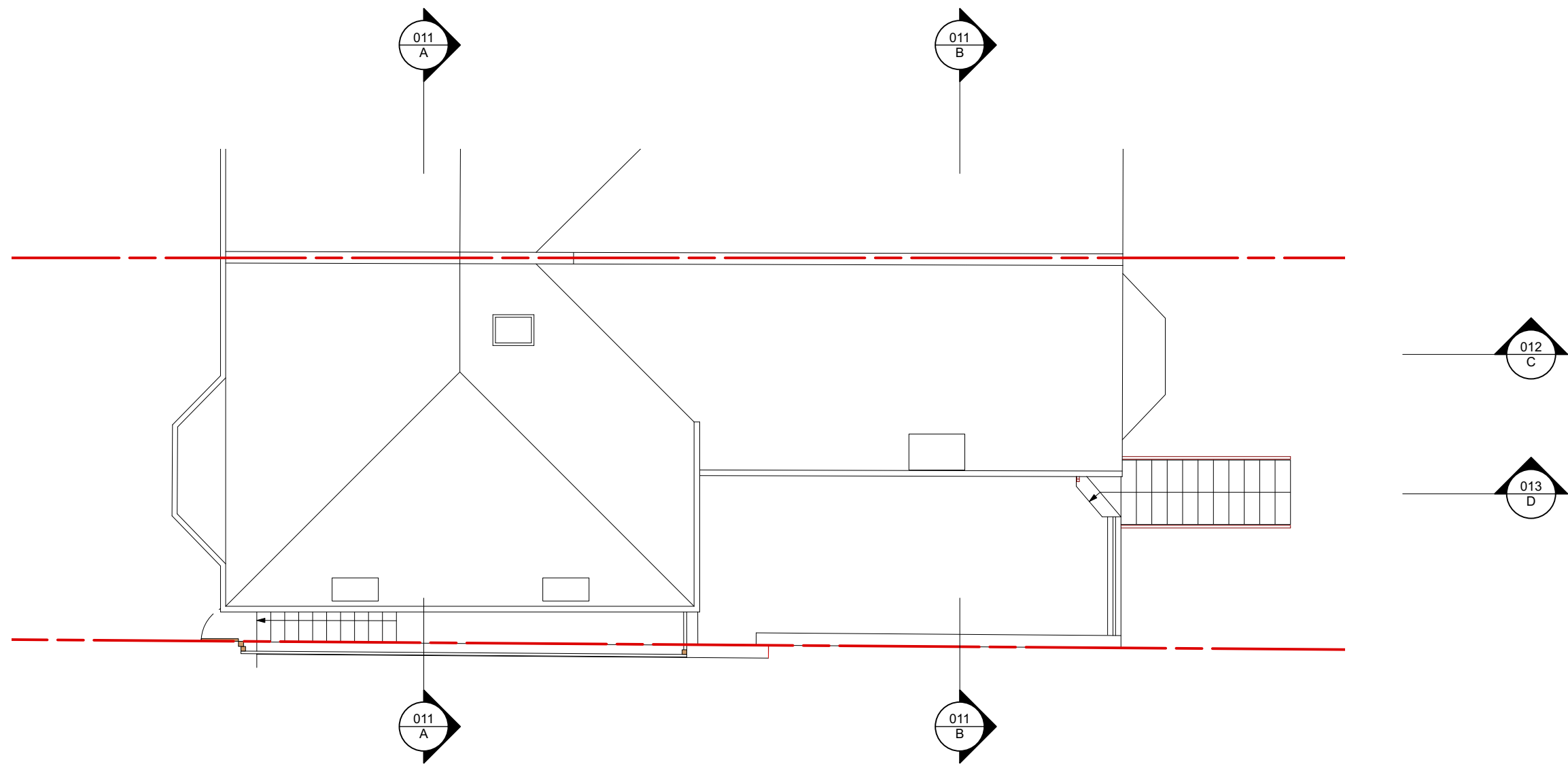
004 Existing Roof Plan Scale: 1:100
