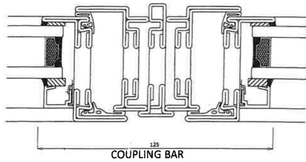
COUPLING BAR
