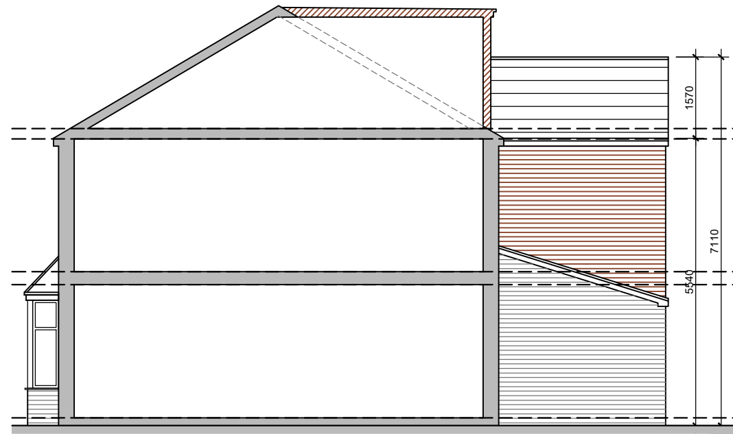
RIGHT ELEVATION
