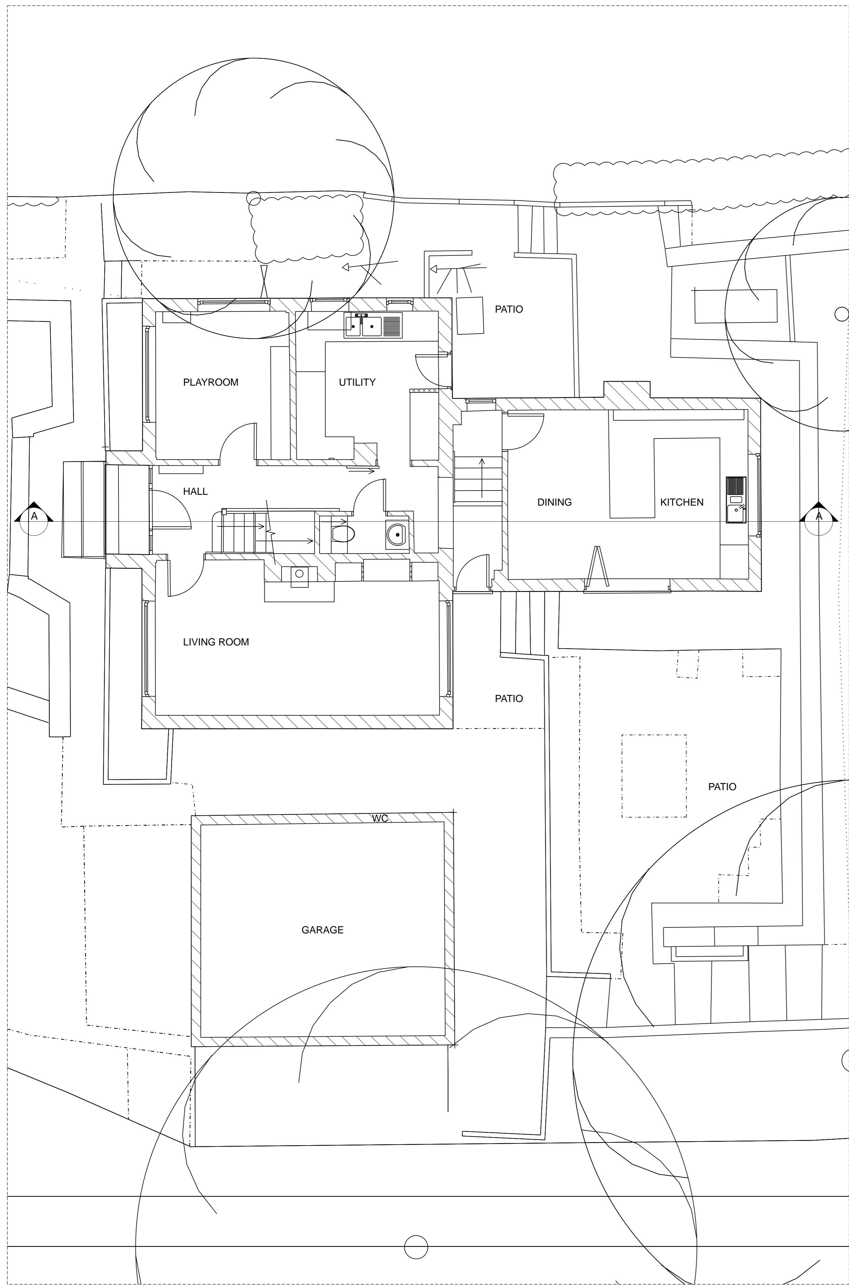
1 EXISTING GROUND Scale: 1:50
