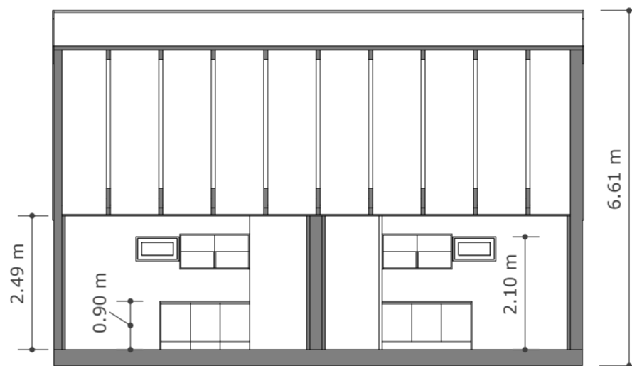
Y A2 SECTION X-X 1:100
