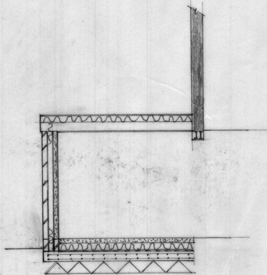
SECTION A-A
