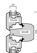
TRANSOM
