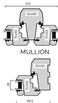
JAMB
