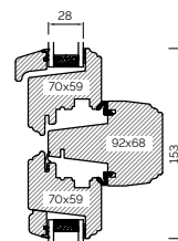
TRANSOM
