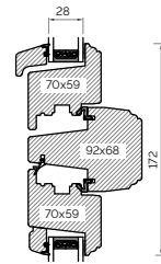
TRANSOM
