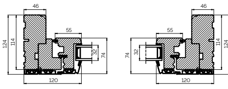
JAMB
