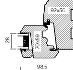
JAMB
