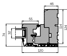
JAMB
