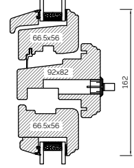
TRANSOM
