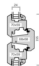
TRANSOM
