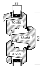
TRANSOM
