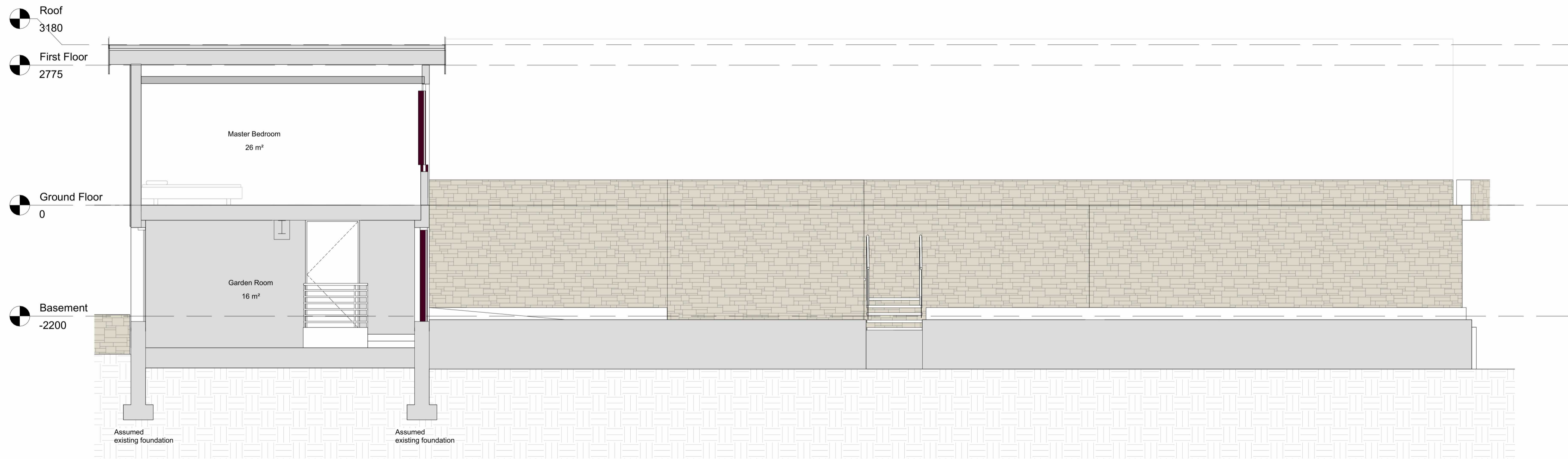
B Existing Section B 1 : 50
