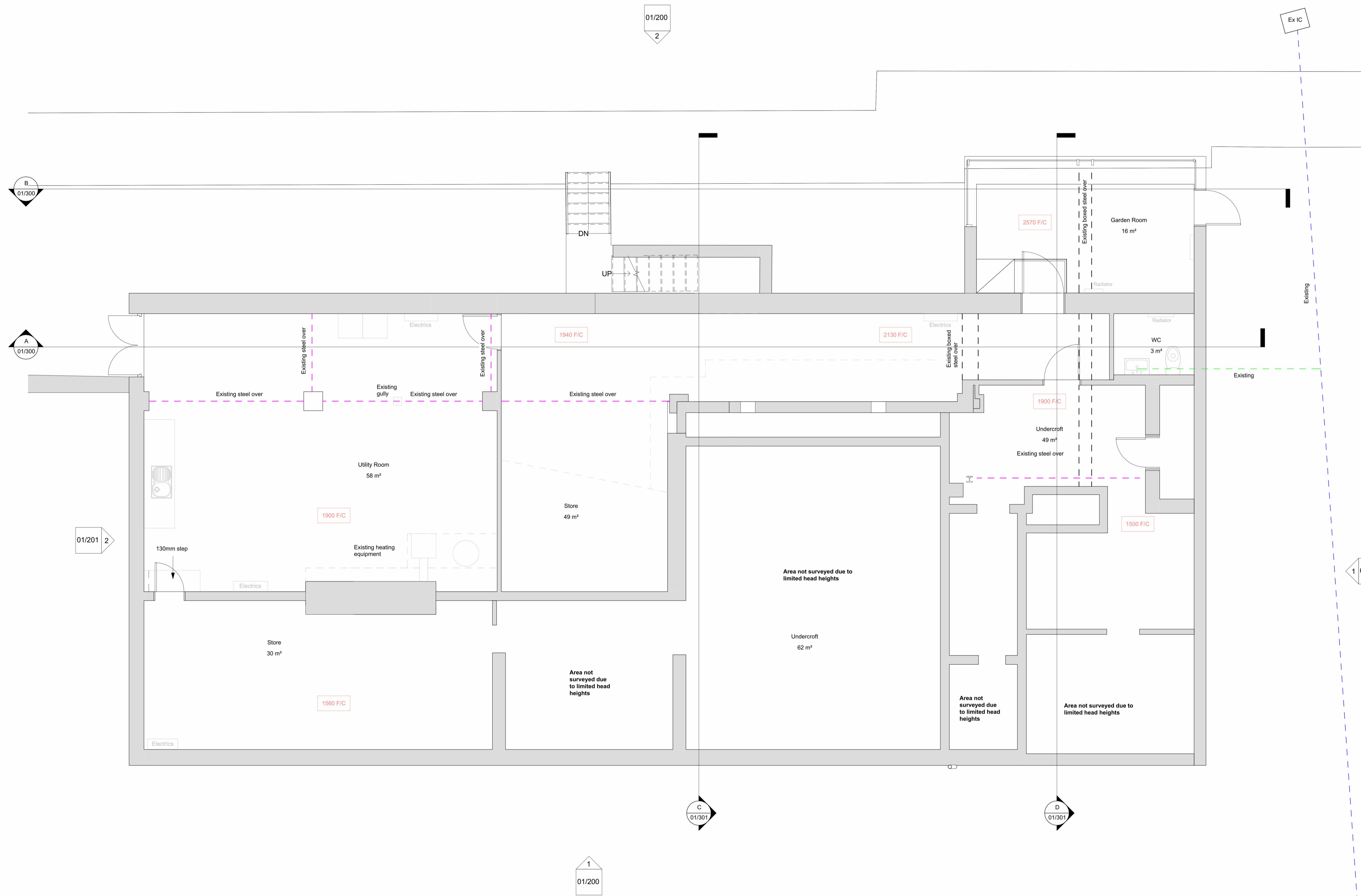
1 Existing Basement 1 : 50
