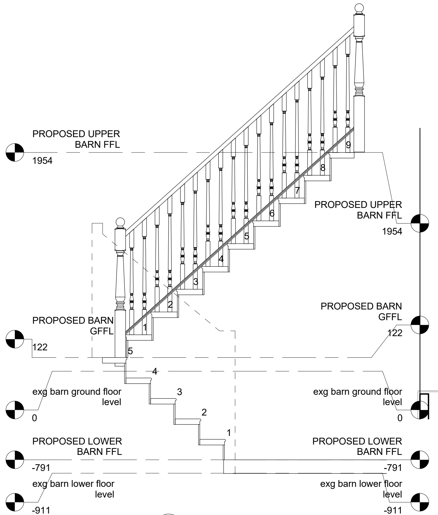
1 STAIR CROSS SECTION 1 : 20
