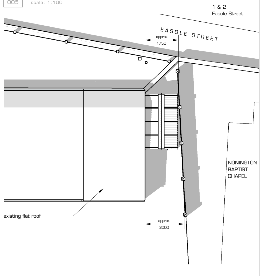
g roof plan 007 scale: 1:100
