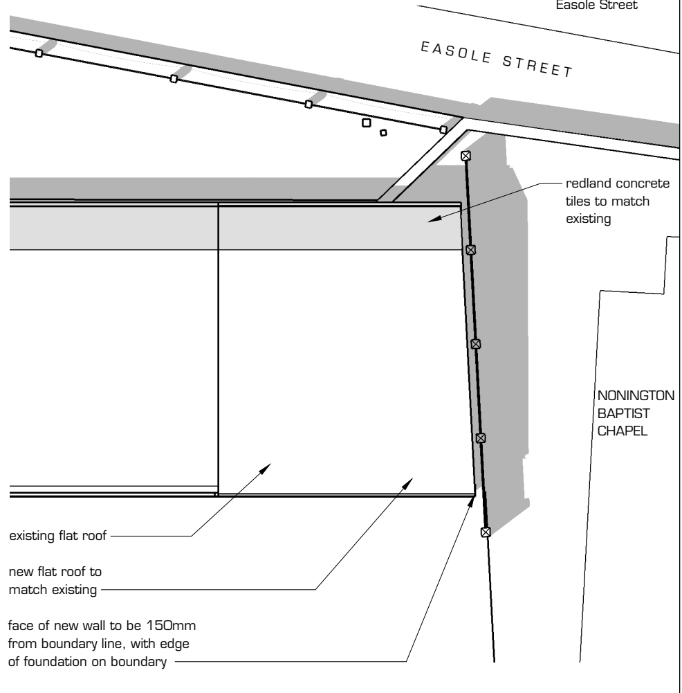
g roof plan 007 scale: 1:100
