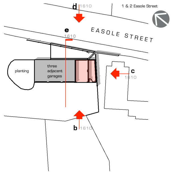
a key plan 001 scale: 1:500
