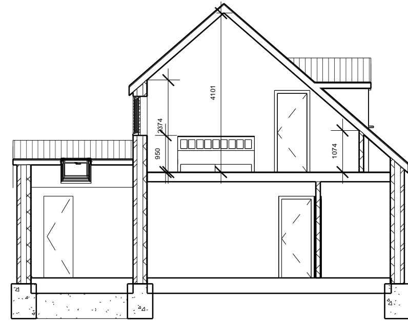
3 Section 1 1 : 100
