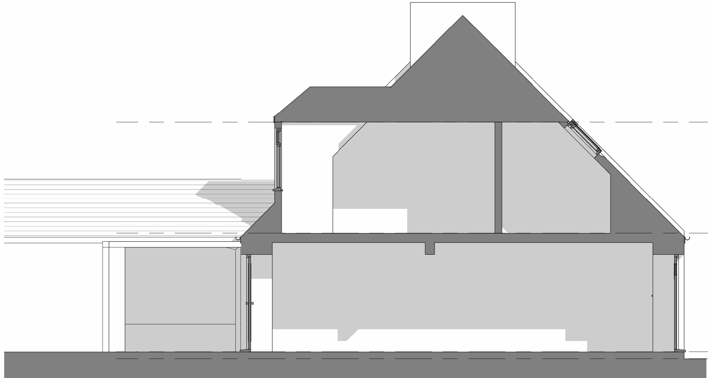
Existing Section AA 1 : 50
