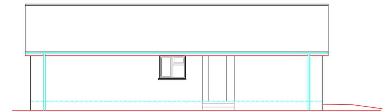
Side SE Elevation
